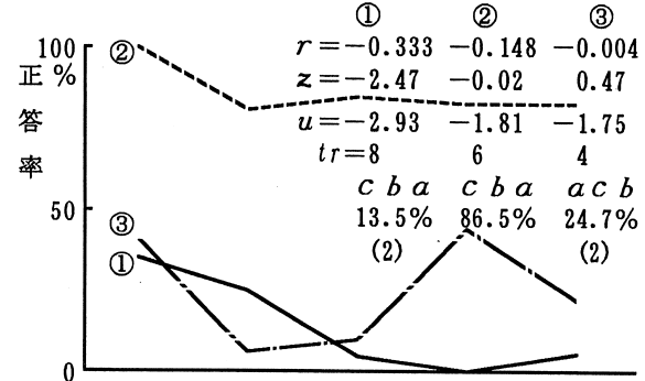
図3-8 uのワースト3 (00)
