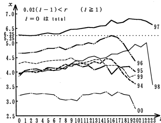
図6 r が条件を満たす問の得点の合格者平均と不合格
