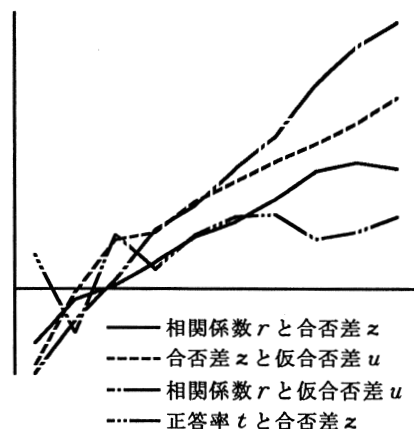
図2-2 合否差( z ), 仮合否差( u ), 相関係数( r ), 正答率( t )の関係 (00)
