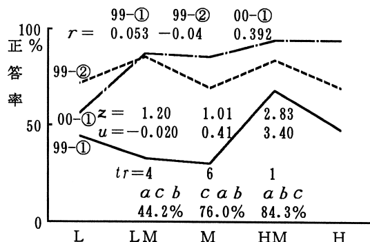
図5 z のワーストの最大比率選択肢を正解と仮定した場合出題者の出張等により正解を確認出来ない問が毎年1~2はある。もう1問は、 z が -1.54 1.16, r が -0.116 0.246, u が -0.52 1.52 と変る。また、99年の z のワーストは、正解とされる選択肢が選ばれた比率が3番目、は2番目である。しかし、とについて、選択された比率が最高の選択肢を正解としたとき、 z > 1 となるが、 r 及び u の絶対値はともに小さく、 tr = 4, 6 で、決して識別性能が高いとは言えない。
