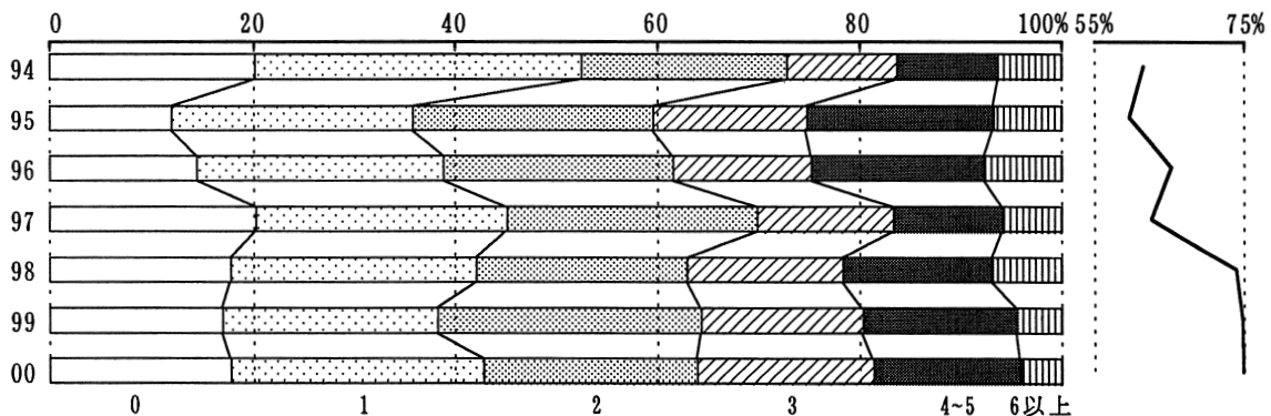
図1 転位数別の問の比率(正答率100%及び0%の問を除く) 平均正答率
