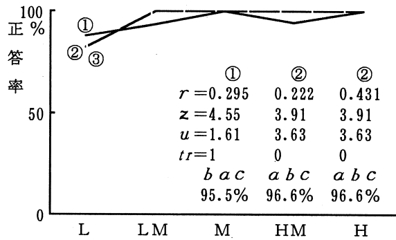
図3-5 zのベスト3 (00)
